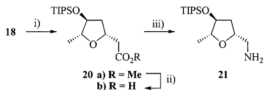
Scheme 2. i) TIPSOTf, 2,6-lutidine, CH 2 Cl 2 , 0^\circ\text{C} , 3 h, 74%; ii) -KOH, MeOH/H 2 O, 20^\circ\text{C} , 16 h, 97%; iii) (PhO) 2 P(O)N 3 , Et 3 N, toluene, 80^\circ\text{C} , 2 h then H 2 O, 20^\circ\text{C} , 16 h, 90%
